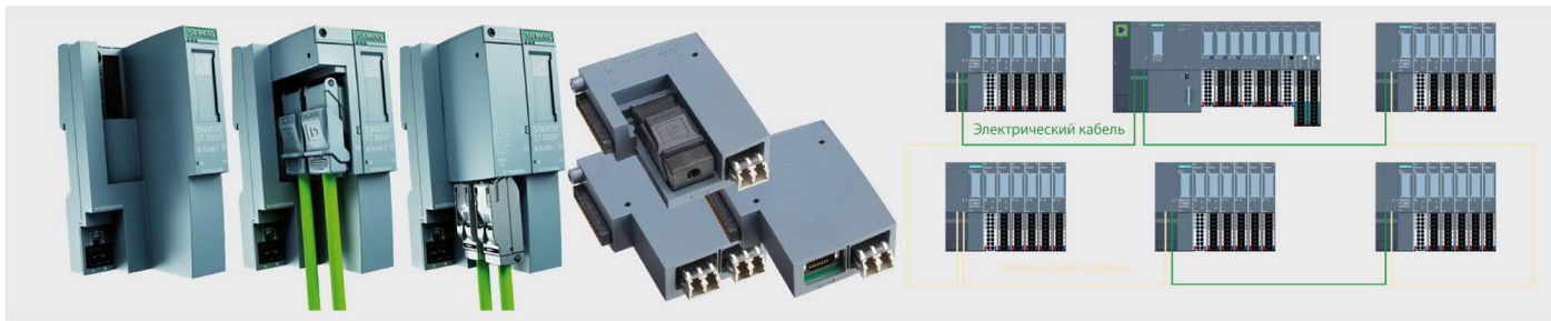
Допустимые варианты установки сетевых адаптеров на модули ET 200SP
